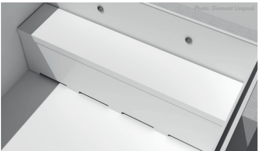
Unterflurschacht einfach (abnehmbare Sitzfläche und Abschirmplatte)
