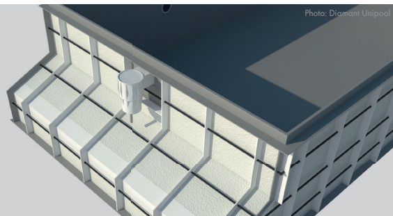
Unterbauschacht für Rollladenabdeckung (inkl. Abschirmplatte)
